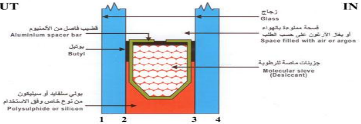
Insulating Glass الزجاج المزدوج العازل
